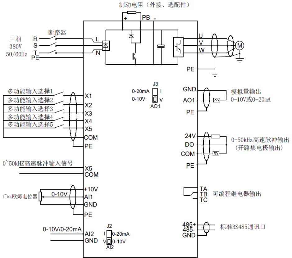
图 2-6 接线图
