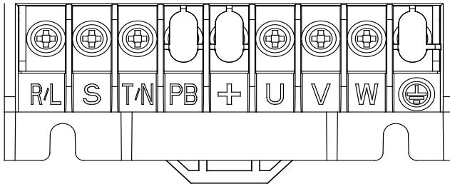
图 2-3 1/3PH 220/380V 0.75-2.2kW 主回路端子接线
