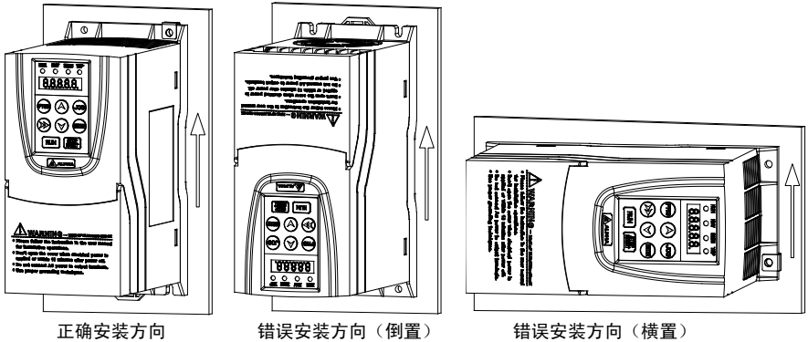
图 2-1 安装方向要求
