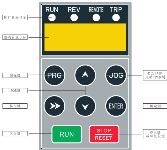
图 3-1 键盘布局与各部分名称
